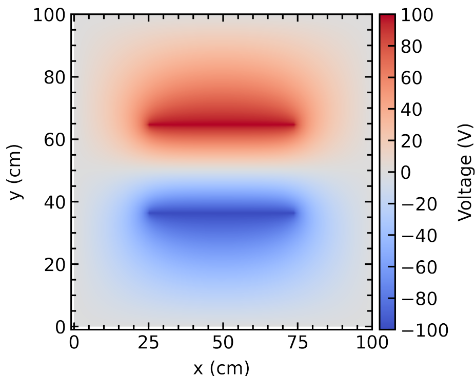
Hình 3: Phân bố thế tĩnh điện cho cấu hình hai thanh song song đối cực, đặt trong hộp vuông nối đất. Đỏ: điện thế dương (gần thanh +100 V); xanh: điện thế âm (gần thanh -100 V); trắng: V = 0 .
