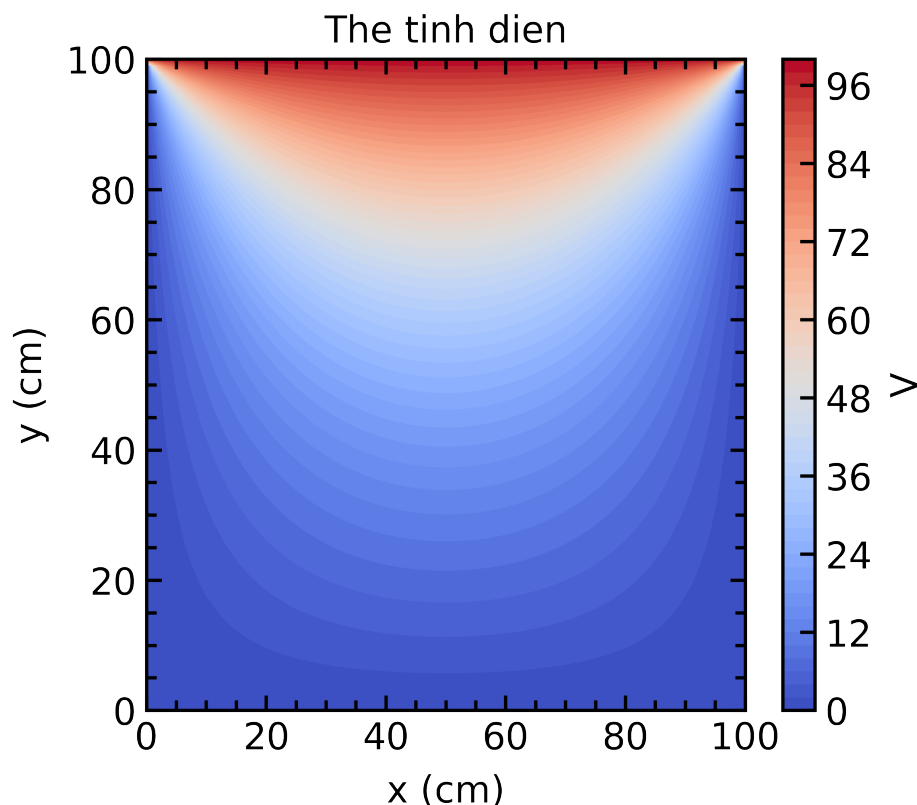
Hình 1: Phân bố thế tĩnh điện V(x, y) trong hình vuông 100 \times 100 \text{ cm} với cạnh trên ở 100 V, ba cạnh còn lại nối đất. Màu đỏ ứng với điện thế cao, màu xanh ứng với điện thế thấp.
